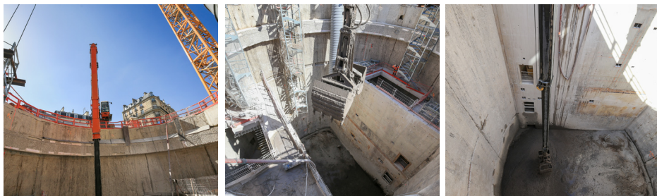
Les travaux de terrassement du Puits Gouraud, juin 2020 © Direction Projet Eole - SNCF Réseau
